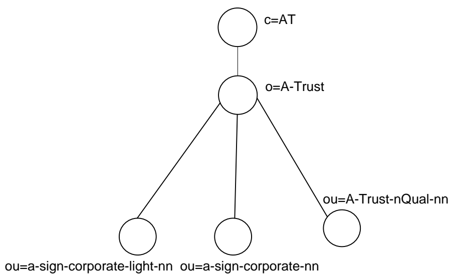
Abbildung 2 a.trust Verzeichnisbaum
