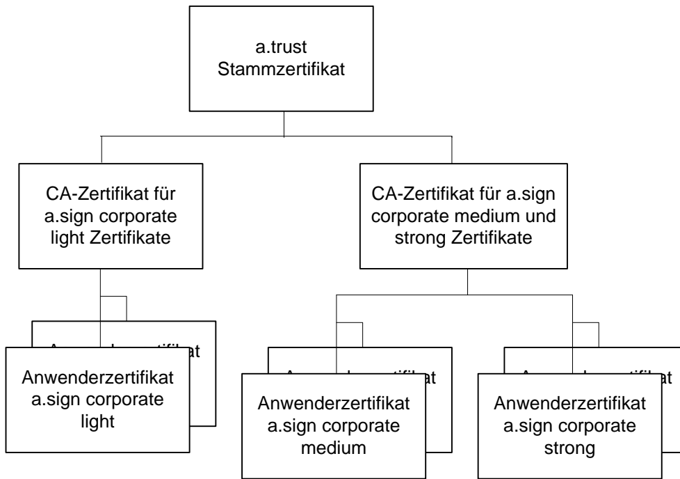
Abbildung 1 Zertifizierungshierarchie
